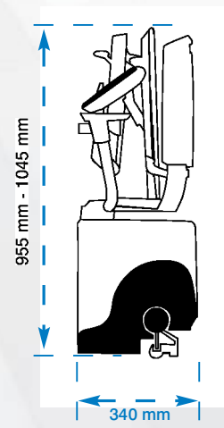
SEITENANSICHT – Zusammengeklappt
