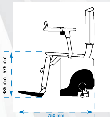
SEITENANSICHT – Aufgeklappt
